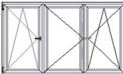
középfelnyíló bukó-nyíló+ bukó-nyíló ablak
